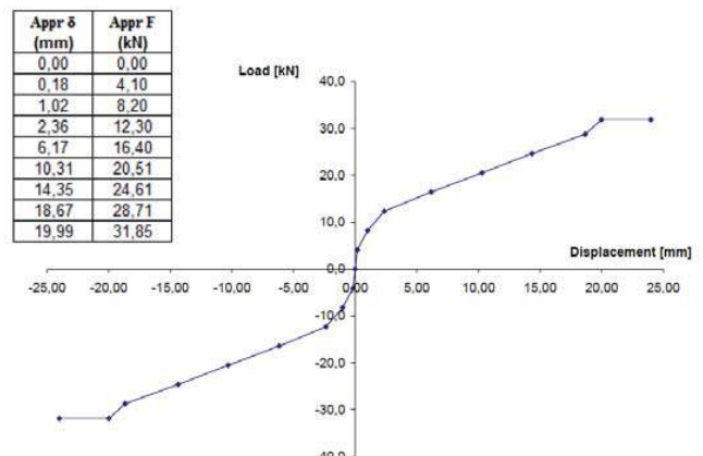
Tvärkraftsstyvhet i horisontalled, V_{y,d}
