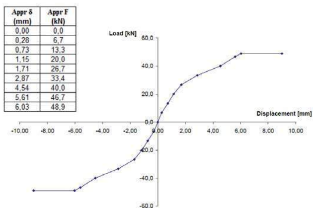
Tvärkraftsstyvhet i vertikalled, V_{z,d}
