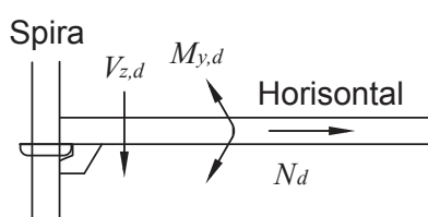
Momentstyvhet i vertikalled, M_{y,d}
