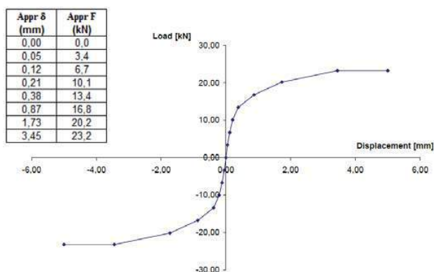
Normalkraftsstyvhet i horisontalled, N_d
