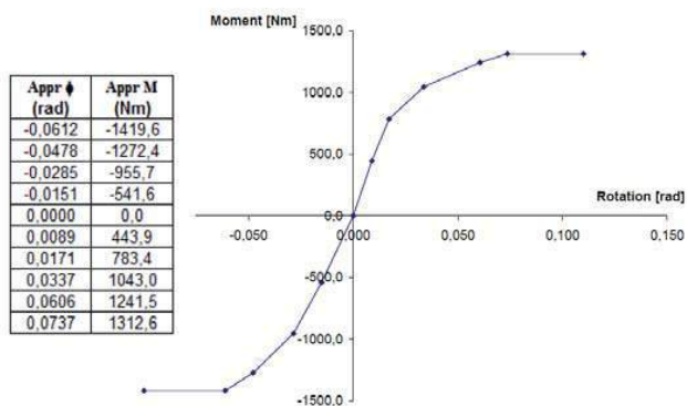
Momentstyvhet i vertikalled, M_{y,d}
